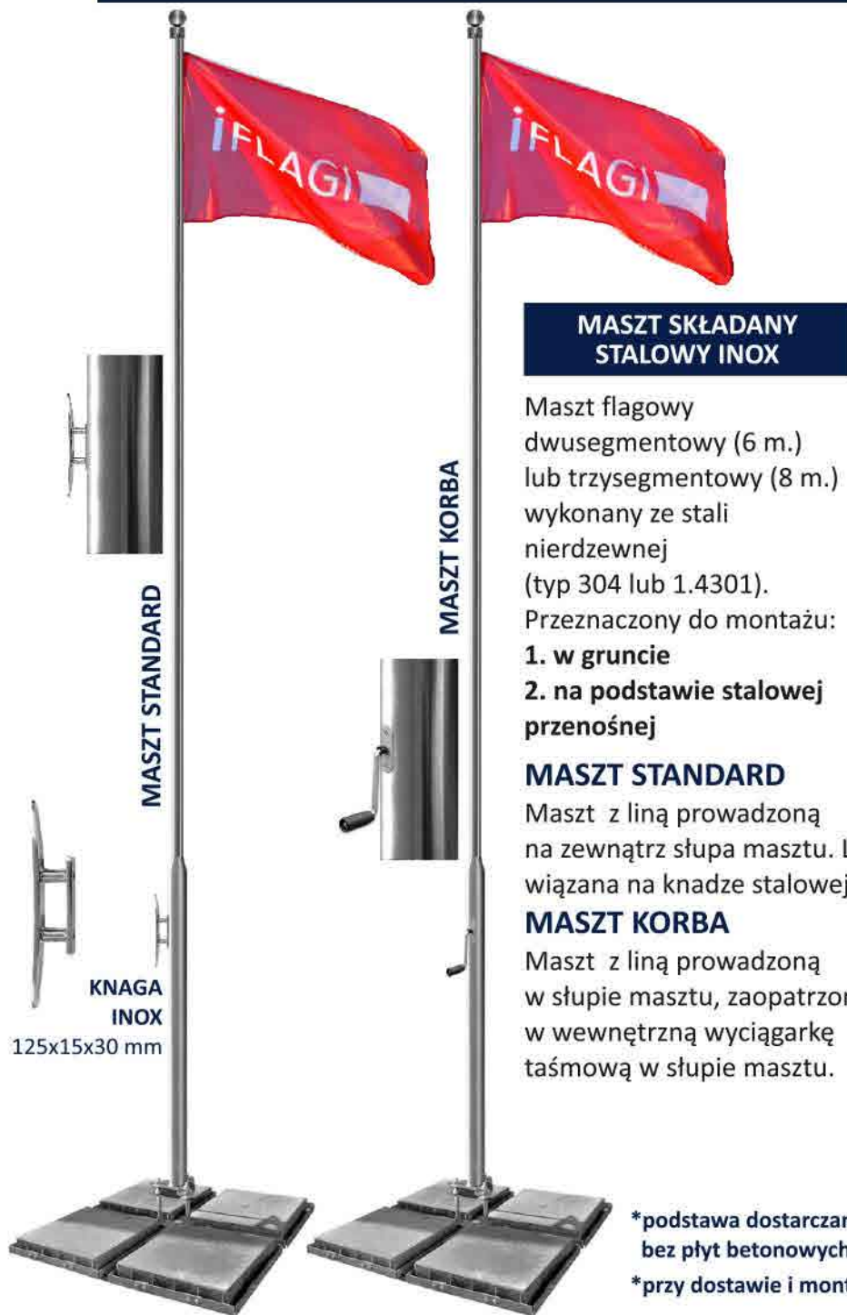
głowica Ø KULA - 10 cm
